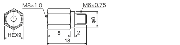
SAG4-6B
