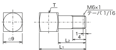
ECMG-6AL, ECMG-6ALL
