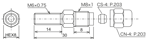
SATG-6B
